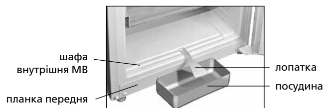
Рисунок 7 – Сбір талої води з МВ
