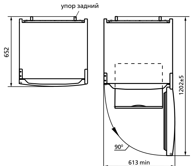
Рисунок 2 – Холодильник (вид сверху)
