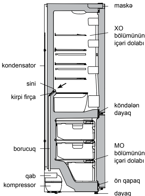
Resim 6 – XO bölümünün ərmiş axıntı sularının tökülmesi sxemi
