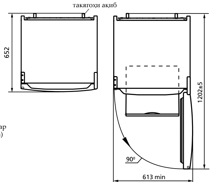
Расми 2 – Яхдон (намуди он аз боло)
