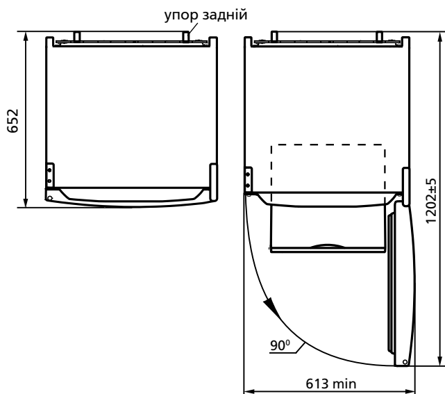
Рисунок 2 – Холодильник (вид зверху)
