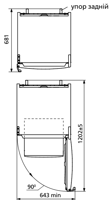
Рисунок 2 – Холодильник (вигляд зверху)
