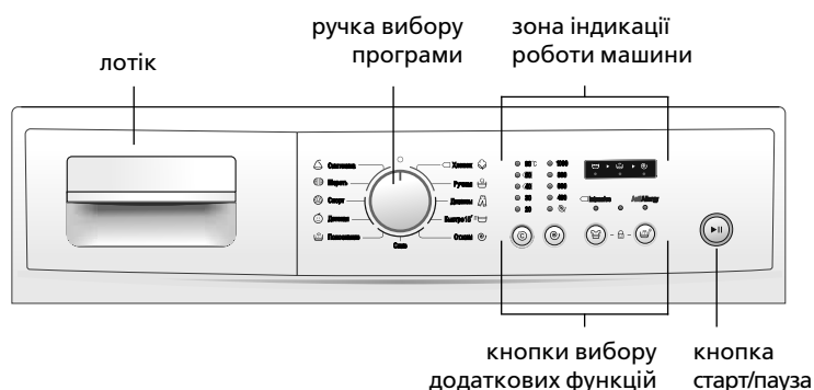
Рисунок 1 – Панель керування
